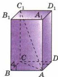
Прямоугольный параллелепипед
