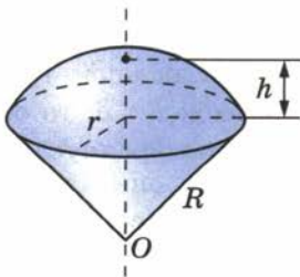
Шаровой сектор
