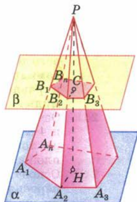
Усеченная пирамида
